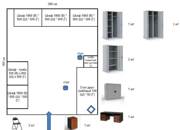
МОДУЛЬ ОХРАНЫ (ОСНАЩЕН ДВЕРЬЮ С ДОВОДЧИКОМ, СТЕКЛОПАКЕТАМИ С ОТКРЫВАЮЩИМИСЯ ОКНАМИ, ЖАЛЮЗИЛИ ИЛИ РУЛОННЫМИ ШТОРАМИ, ДЕКОРАТИВНОЙ ПОДСВЕТКОЙ)
